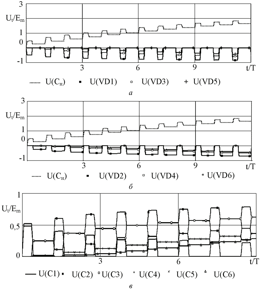
Рисунок 3 – Напряжения на элементах схемы при несимметричном виде источника E : a , б – напряжения на диодах; в – напряжения на конденсаторах
