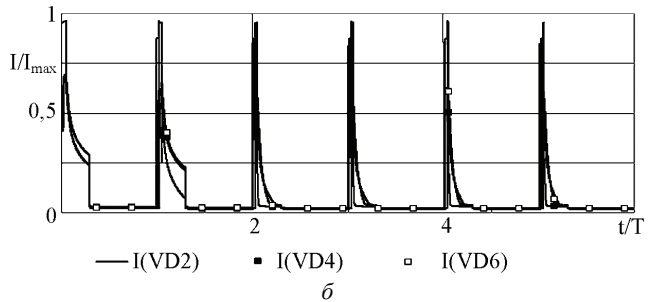
Рисунок 5 – Токи через диоды при несимметричной виде источника E: a – токи через диоды VD1,VD3,VD5; b – токи через диоды VD2,VD4,VD6
