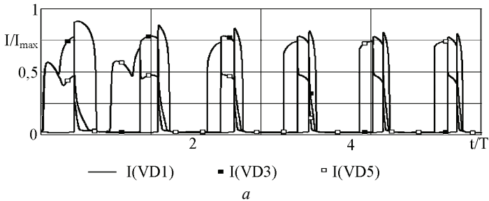
Рисунок 5 – Токи через диоды при несимметричной виде источника E: a – токи через диоды VD1,VD3,VD5; b – токи через диоды VD2,VD4,VD6
