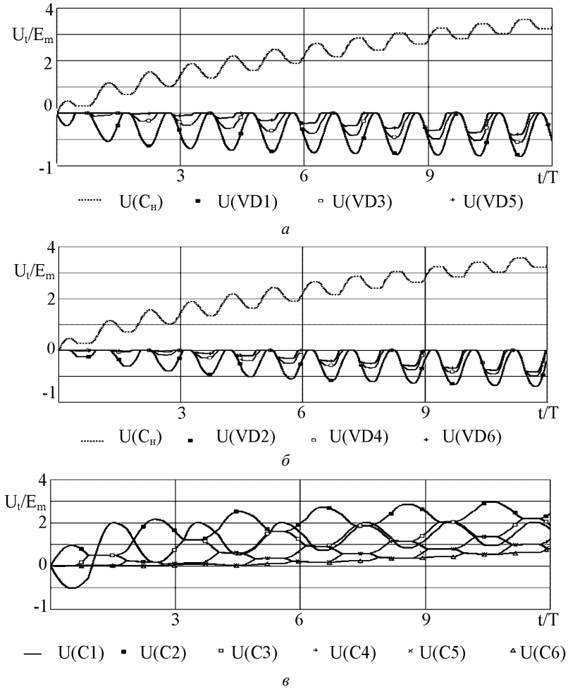
Рисунок 4 – Напряжения на элементах схемы при симметричном виде источника E: а, б – напряжения на диодах; в – напряжения на конденсаторах
