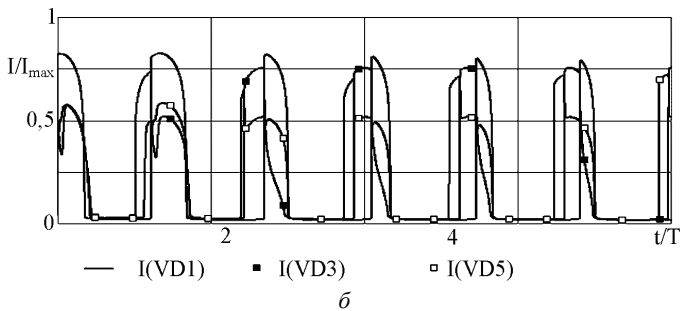
Рисунок 6 – Токи через диоды при симметричной виде источника E: a – токи через диоды VD1,VD3,VD5; b – токи через диоды VD2,VD4,VD6
